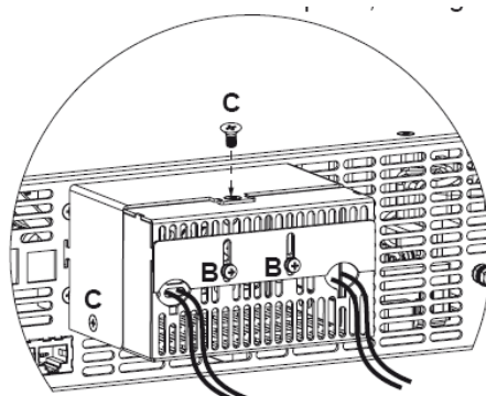
*поставка для моделей выпуска 2016г и после Рис.3-10: Сборка защитного кожуха и проводов
