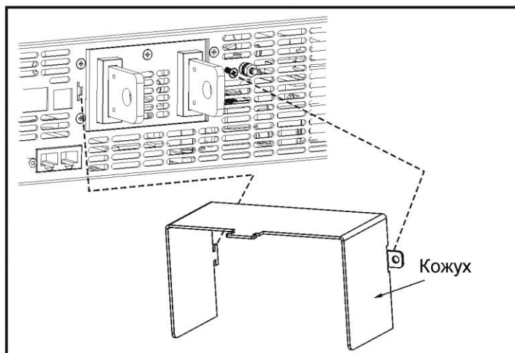
Рис. 3-7: Монтаж кожуха
