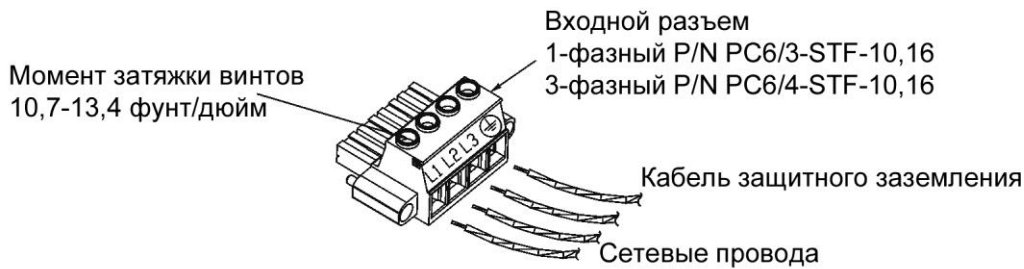
Рис.3-3: Входной разъем (на рисунке трехфазный)
